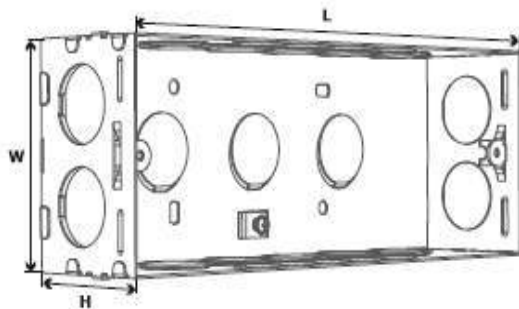
8 MODULE (SQ)
